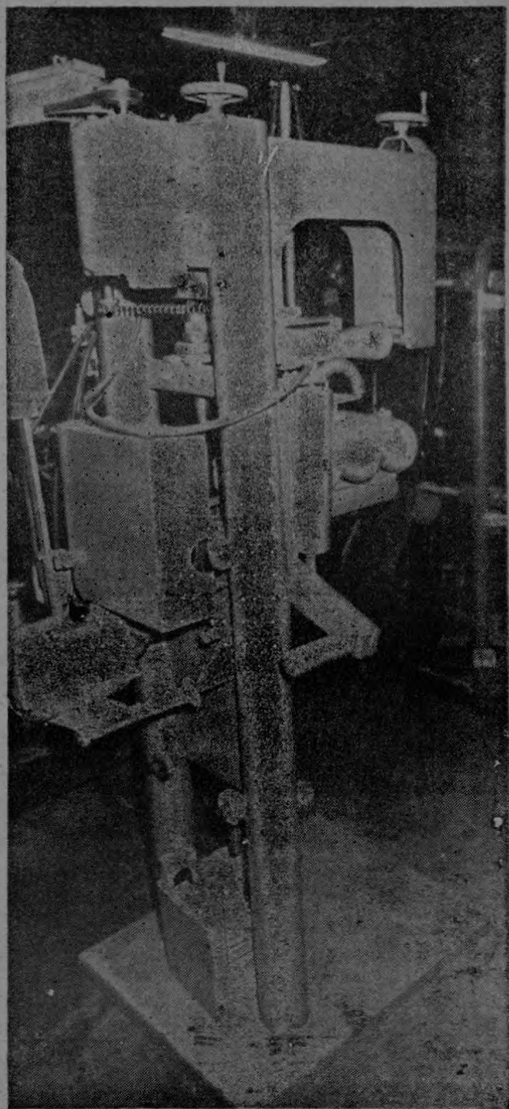
EM BANDADORA SEMIAUTOMATICA para embandar con rapidez y precisión las llantas para ser recauchadas.
