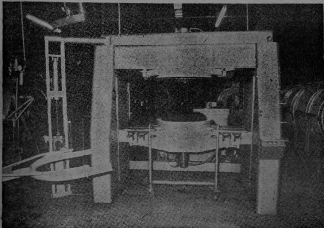
PRENSA LODI-ELECTRA II, la cual automáticamente coloca la llanta en el molde y la deja perfectamente ajustada e instalada para el proceso de vulcanización.
