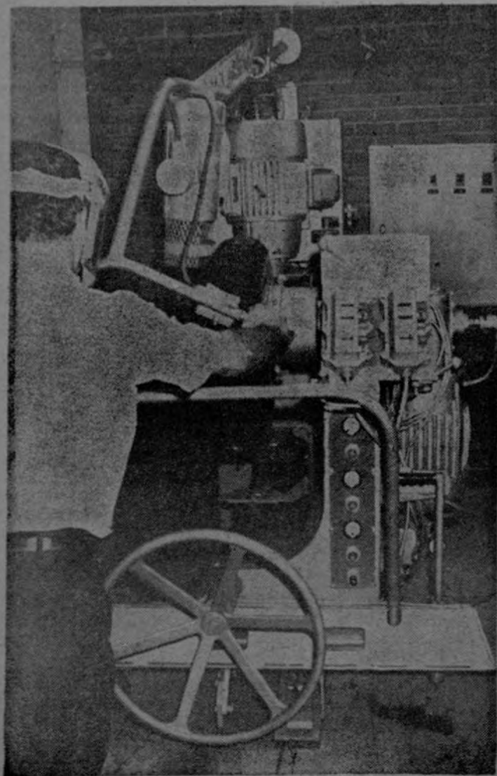
RASPADOR DE LLANTAS - Modelo Lodi BU - 2, se utiliza para el proceso de raspado.
